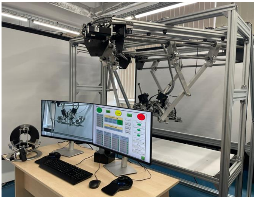
Sistem modular cu 3 grade de libertate cu constrângerea mecanică a RCM-ului (CESTER)
